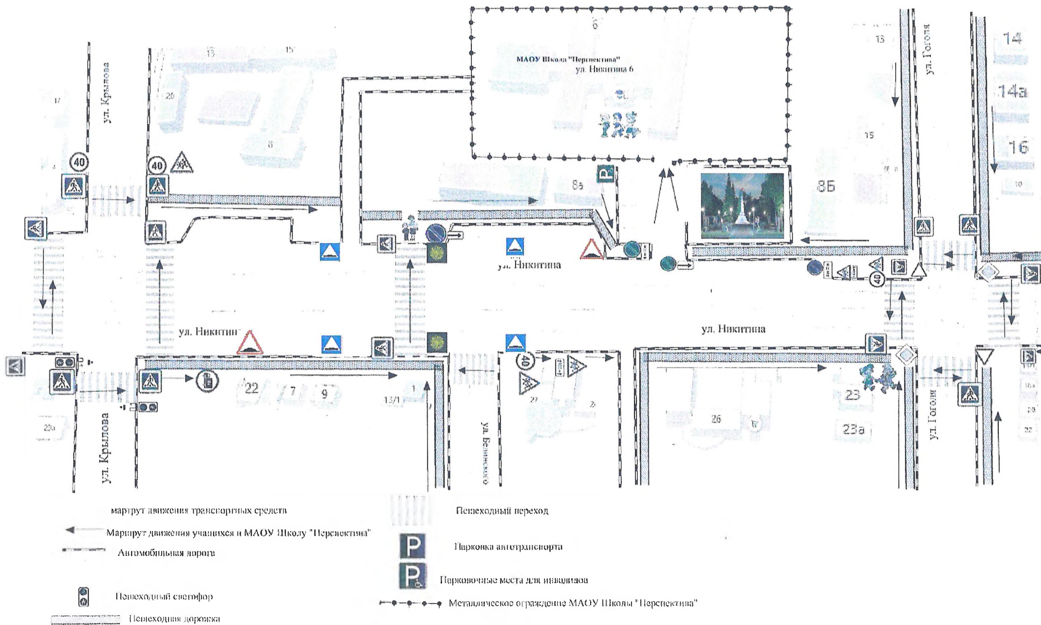
Схема организации дорожного движения в непосредственной близости от образовательной организации с размещением соответствующих технических средств организации дорожного движения, маршрутов движения детей и расположение парковочных мест.
